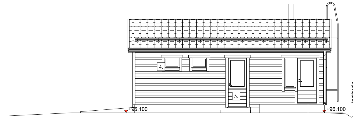
JULKISIVU ITÄÄN
