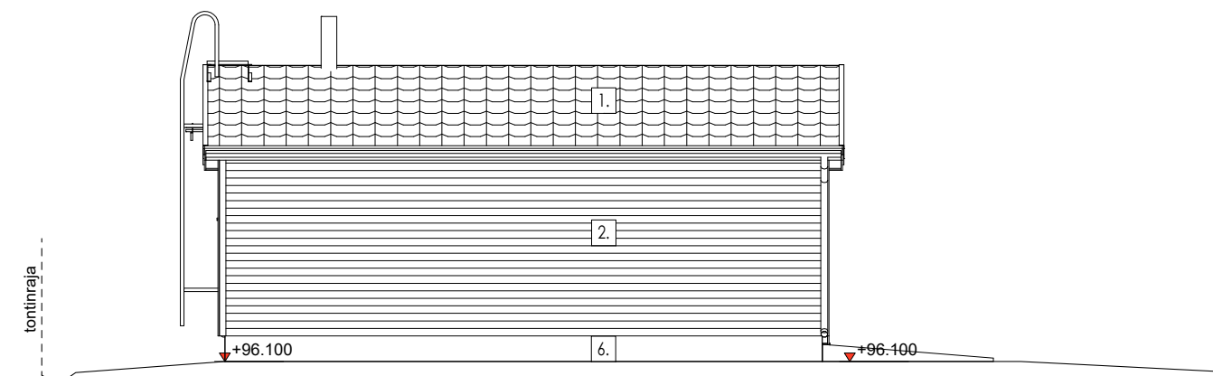
JULKISIVU LÄNTEEN
