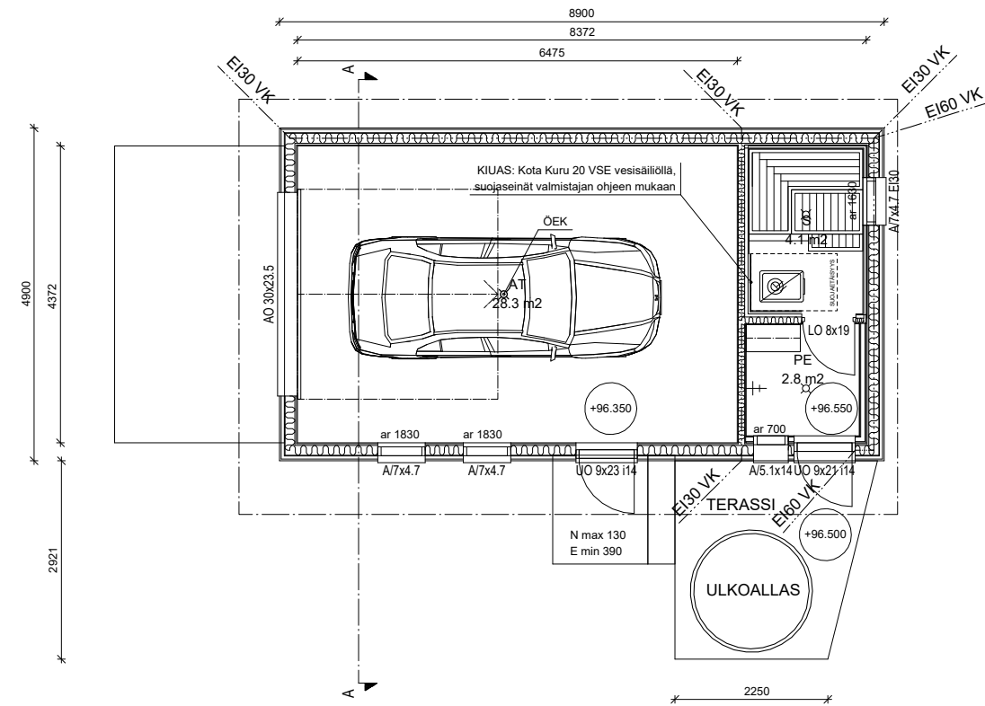
HORMISTO 1:20
