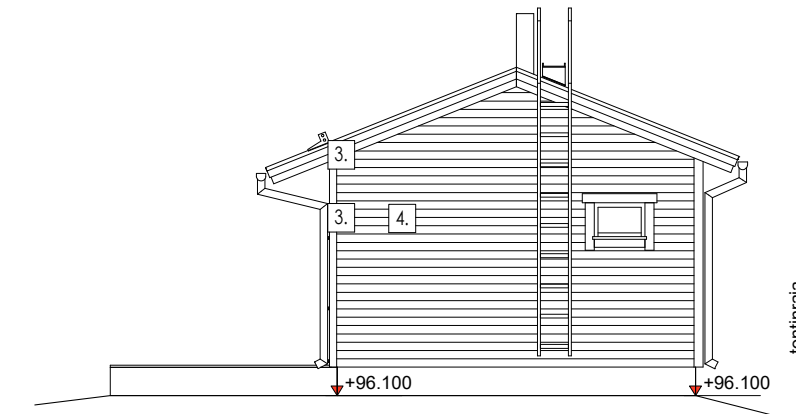
JULKISIVU POHJOISEN
