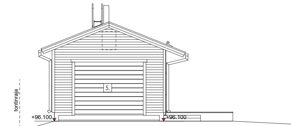
JULKISIVU ETELÄÄN
